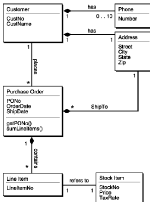
Рис. 2. Диаграмма классов предметной области «Заказы»
