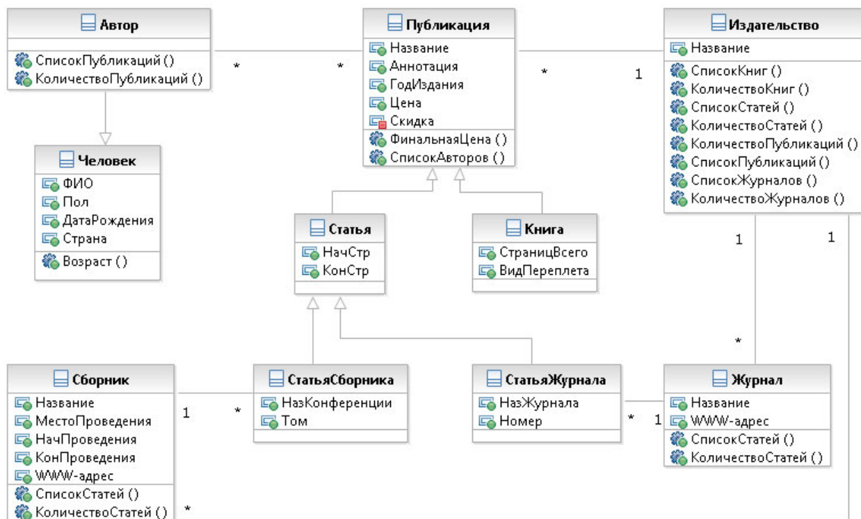
Рис. 1. Диаграмма классов предметной области «Интернет магазин научных публикаций»
