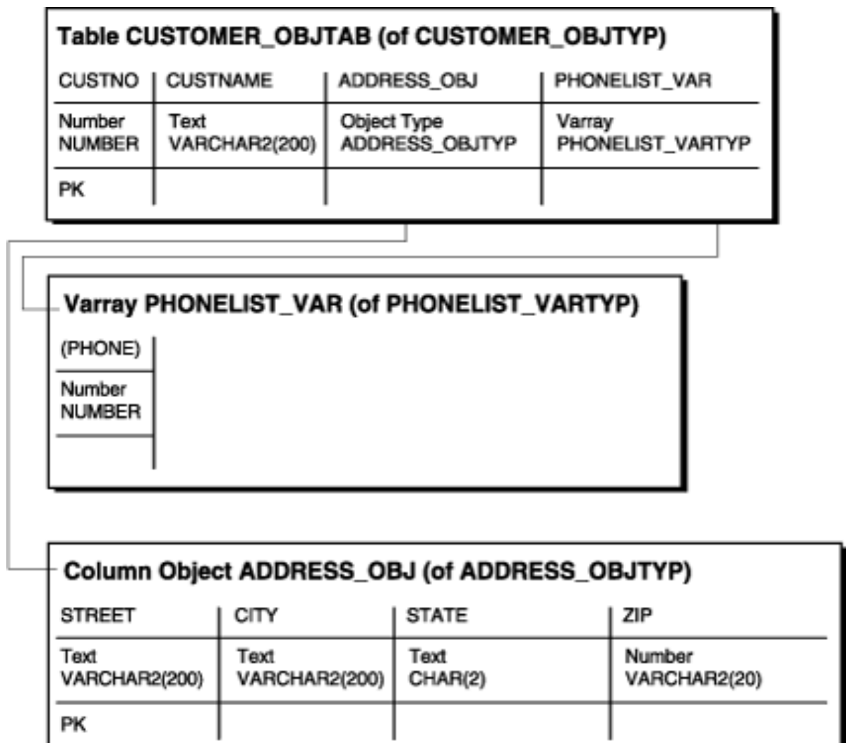
Рис. 4. Объектно-реляционное представление таблицы Customer_objtab
