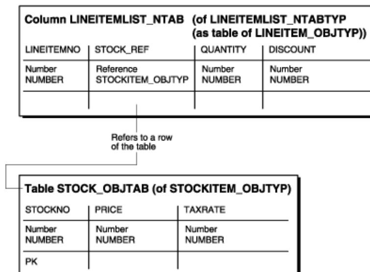
Рис. 6. Объектно-реляционное представление таблицы LineItemList_ntab
