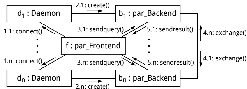
Рис. 7. Взаимодействие клиента и серверов PargreSQL
